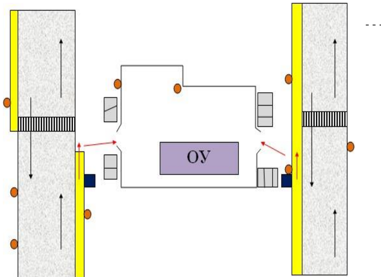
Схема 2. Схема организации дорожного движения в непосредственной близости от образовательного учреждения с размещением соответствующих технических средств организации дорожного движения, маршрутов движения детей (обучающихся, воспитанников) и расположения парковочных мест.
